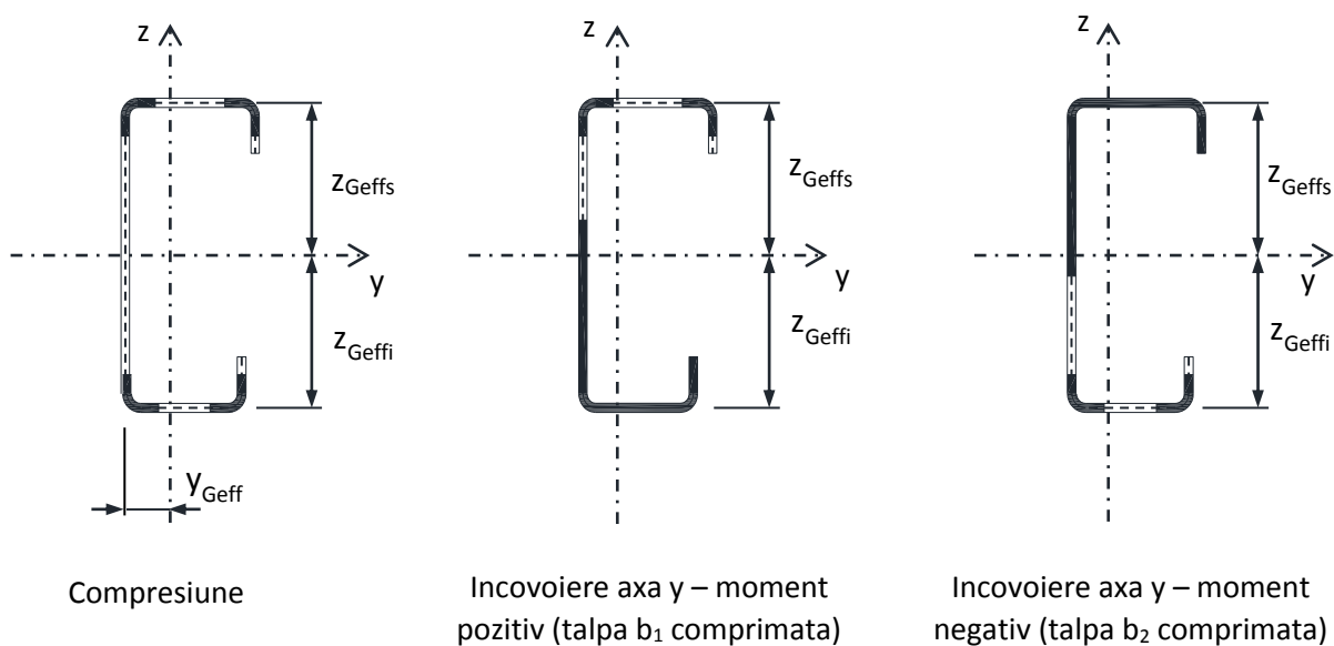
Figura 2 Notatii caracteristici geometrice pentru sectiunile efective de calcul
