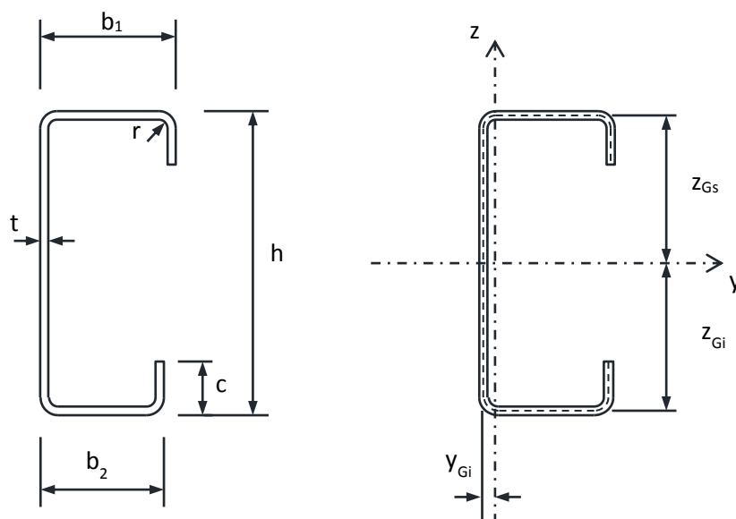
Figura 1. Notatii dimensiuni profile Z si caracteristici geometrice pentru sectiunea bruta
