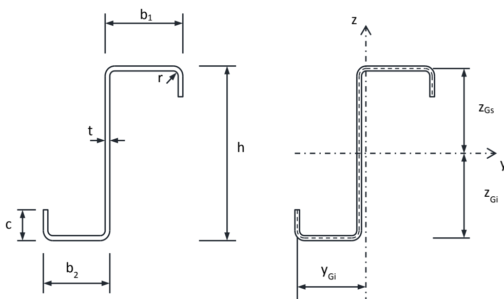
Figura 1. Notatii dimensiuni profile Z si caracteristici geometrice pentru sectiunea bruta
