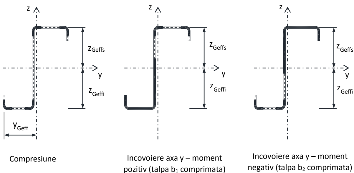
Figura 2 Notatii caracteristici geometrice pentru sectiunile effective de calcul
