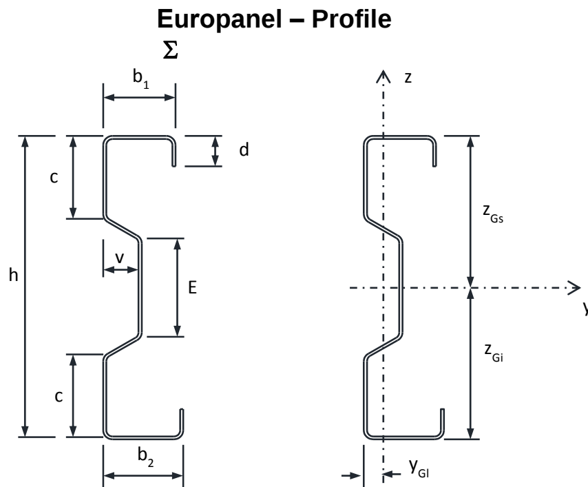
Figura 1. Notatii dimensiuni profile \Sigma si caracteristici geometrice pentru sectiunea bruta
