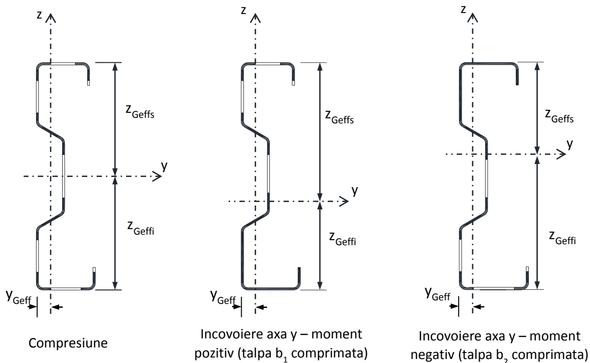
Figura 2 Notatii caracteristici geometrice pentru sectiunile efective de calcul
